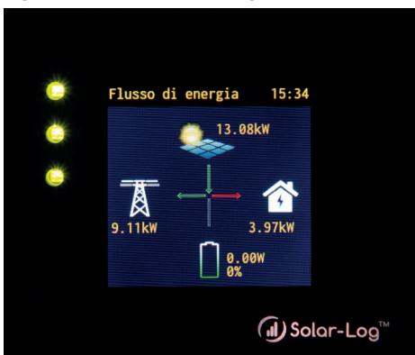
Fig.: Esempio impianto con flusso di energia
